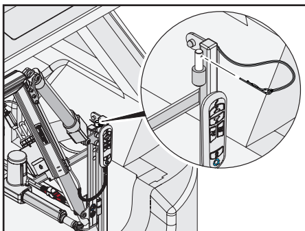
4. Nasaďte R-klip na horní kolík rámu.
