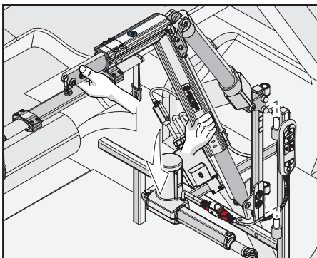
2. Spusťte zvedák L-P na dva kolíky podle pokynů. Ujistěte se, že je zvedák řádně připevněn.
