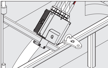
2. Odnímatelný držák motoru na levé straně.
